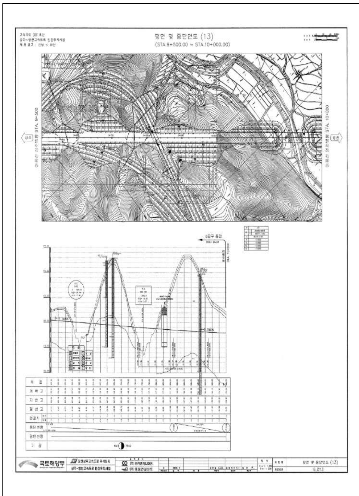
【그림 58.3】 평면도
